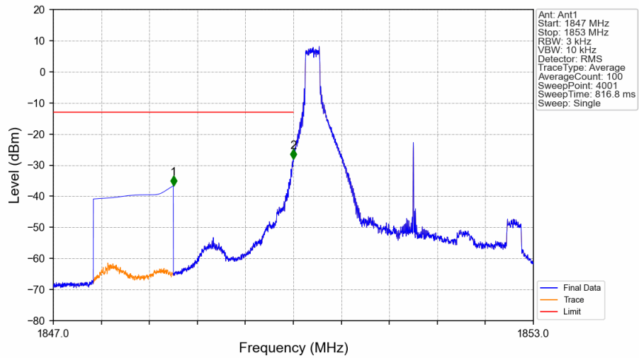
Band2_3MHz_QPSK_LCH_1851.5MHz_RB_1_0_NTNV
