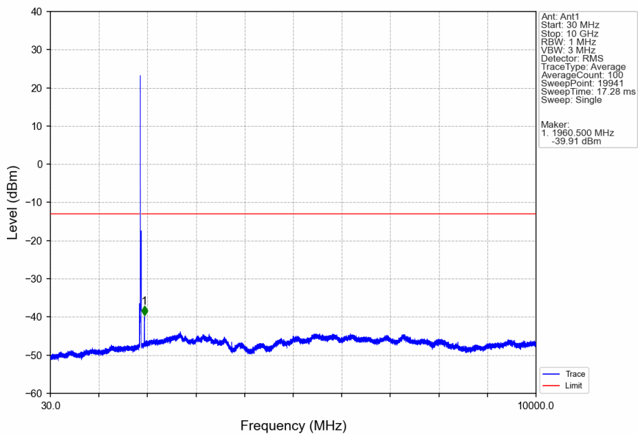
Band2_10MHz_QPSK_MCH_1880MHz_RB_1_0_NTNV
