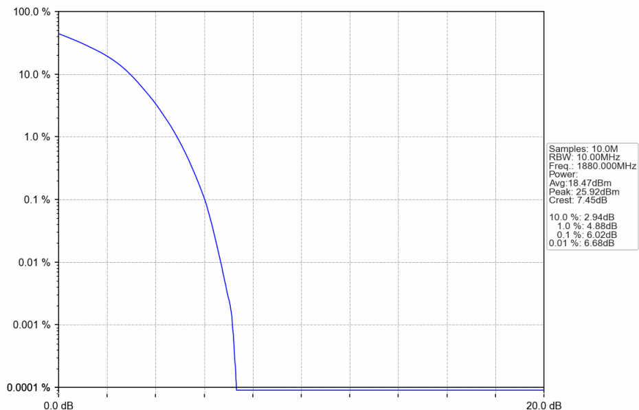
Band2_10MHz_16QAM_MCH_1880MHz_RB_50_0_NTNV
