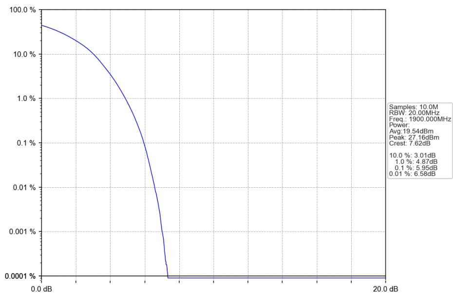
Band2_20MHz_16QAM_HCH_1900MHz_RB_100_0_NTNV
