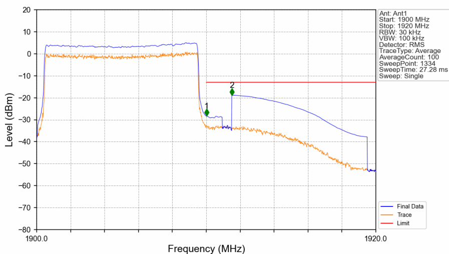
Band2_10MHz_16QAM_HCH_1905MHz_RB_50_0_NTNV
