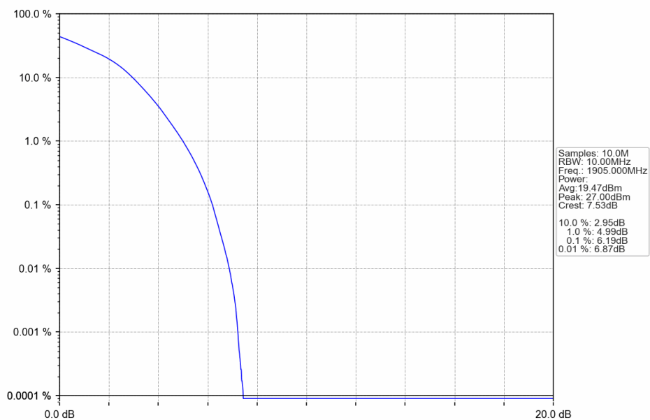
Band2_10MHz_16QAM_HCH_1905MHz_RB_50_0_NTNV
