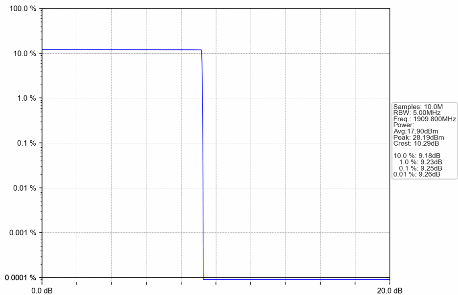
PCS1900 GSM HCH 1909.8MHz GSM NTV
