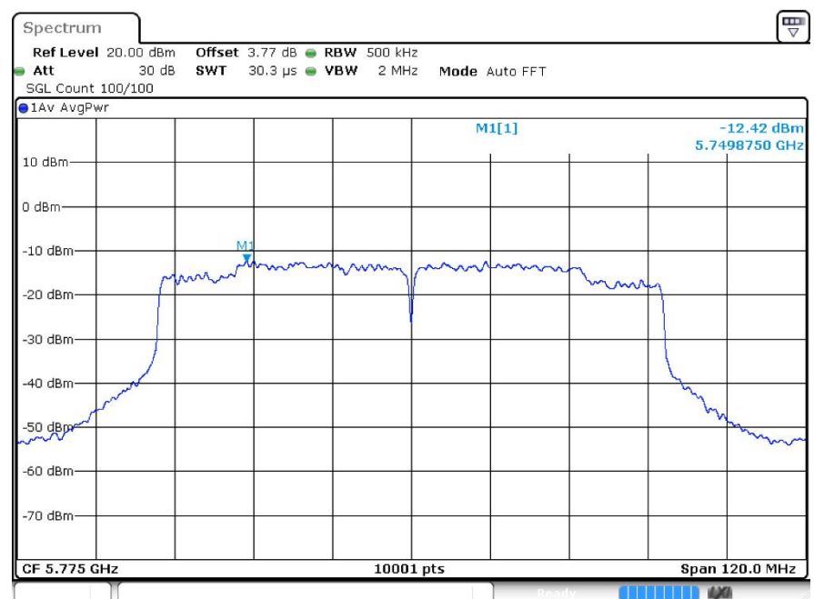
PSD ac80 5775MHz Ant1
