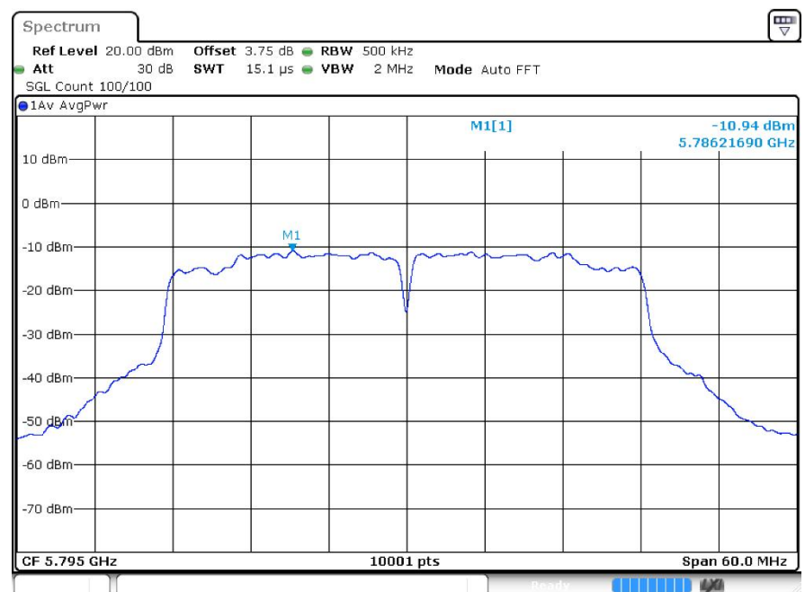
PSD ac40 5795MHz Ant1
