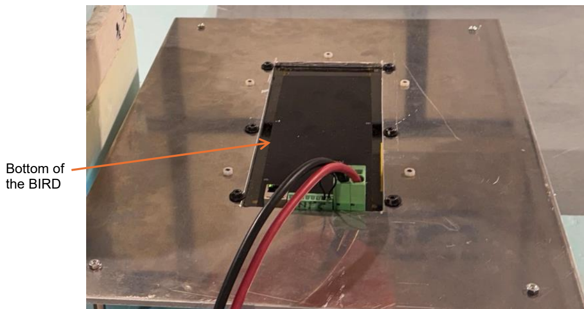
BIRD actual photo of the part – NFC mode
