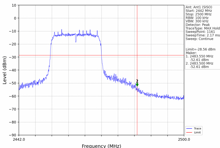
802.11n(HT20)_HCH_2462MHz_Ant1 (SISO)_NTNV
