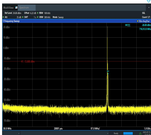
Band12-3MHz-QPSK-23165-1RB#0-30~1000-P ASS
