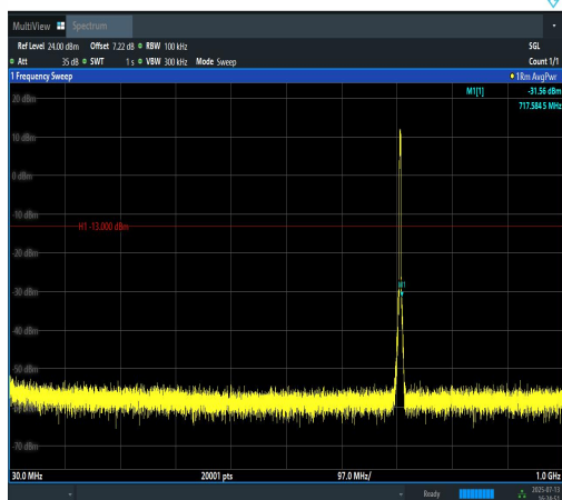
Band12-3MHz-QPSK-23165-15RB#0-30~1000-P ASS
