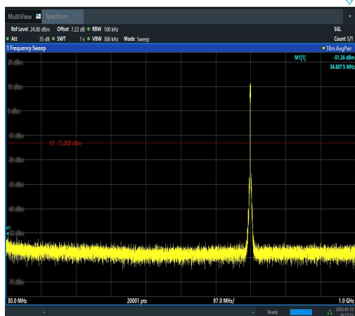
Band12-3MHz-QPSK-23095-15RB#0-30~1000-P ASS
