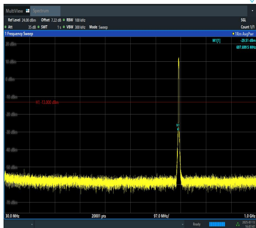
Band12-3MHz-QPSK-23025-15RB#0-30~1000-P ASS
