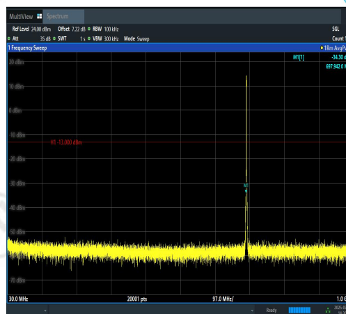
Band12-1.4MHz-16QAM-23017-6RB#0-30~1000- -PASS
