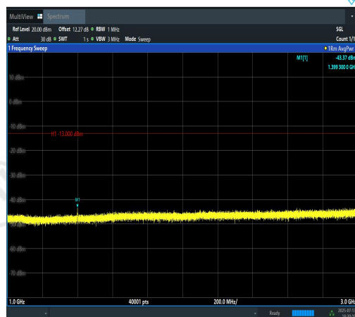
Band12-1.4MHz-QPSK-23017-6RB#0-1000~300 0-PASS
