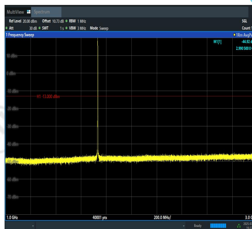
Band4-1.4MHz-QPSK-20175-1RB#0-1000~3000 -PASS
