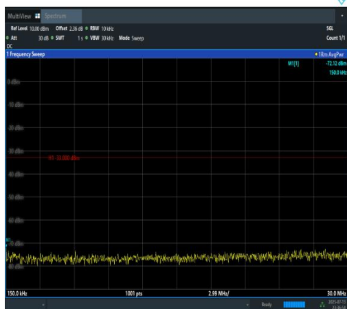
Band2-20MHz-QPSK-18700-1RB#99-0.15~30-P ASS
