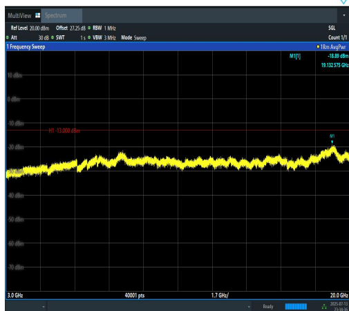
Band2-20MHz-QPSK-18700-1RB#0-3000~2000 0-PASS
