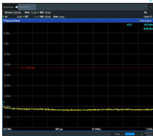
Band2-15MHz-QPSK-19125-1RB#0-30~1000-P ASS
