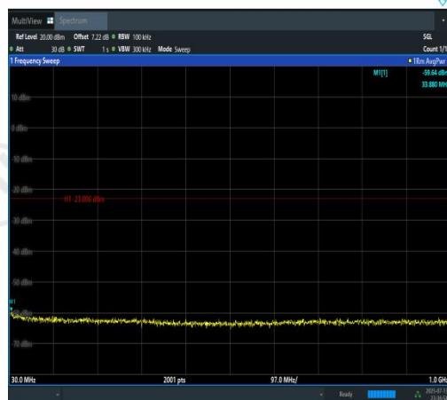
Band2-20MHz-QPSK-18700-1RB#99-30~1000-P ASS
