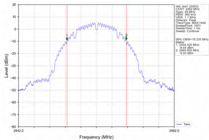
802.11b_HCH_2462MHz_Ant1 (SISO)_NTNV
