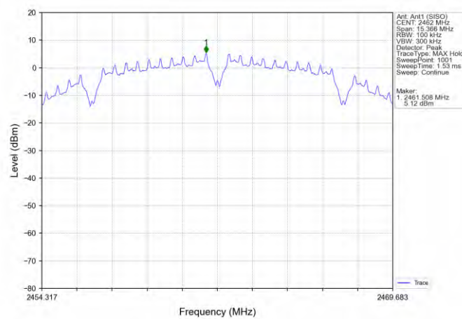
802.11b_HCH_2462MHz_Ant1 (SISO)_NTNV
