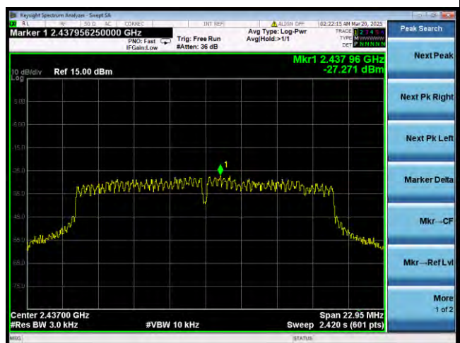
802.11g 2437MHz
