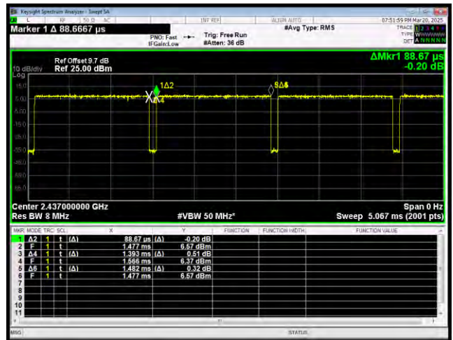
802.11g 2437MHz
