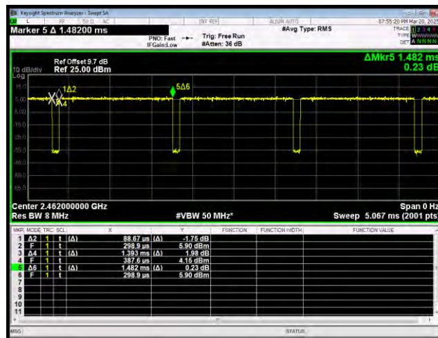
802.11g 2462MHz
