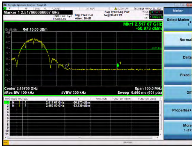
802.11b MHz
