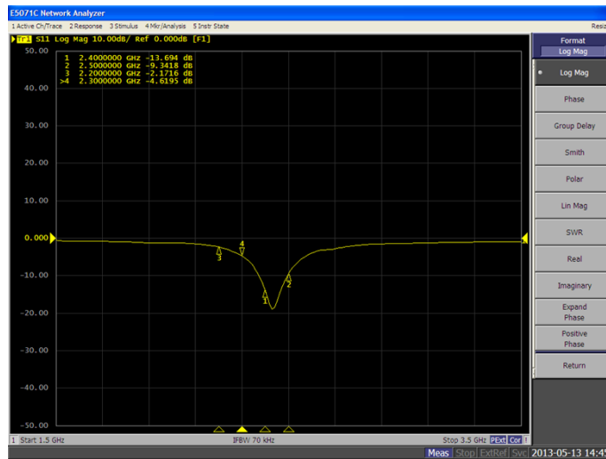
图 3 Antenna S11
