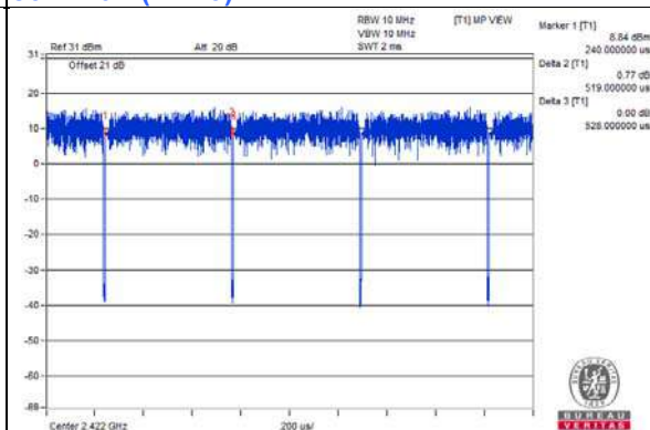
802.11ax (RU52)
