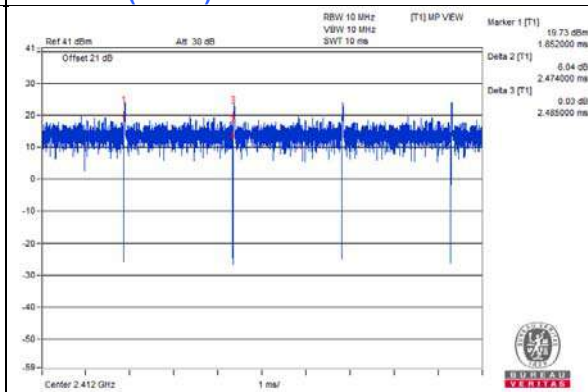
802.11ax (RU52)
