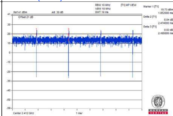
802.11ax (RU52)
