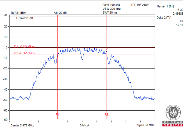
802.11ax (HE20) / Chain 0 : CH13
