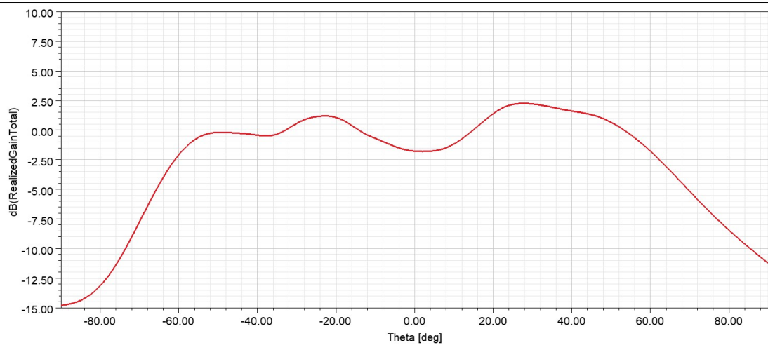
俯仰面方向图 (TX1) Freq: 63. 0GHz
