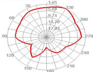
5400.000MHz E2
