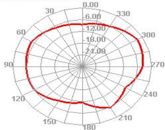
5400.000MHz E2
