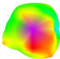
5400.000MHz E1
