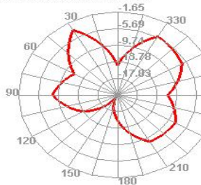
5400.000MHz E1
