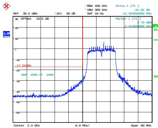
802.11n20_2412MHz
