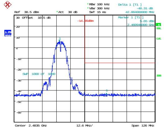
802.11b_2462MHz
