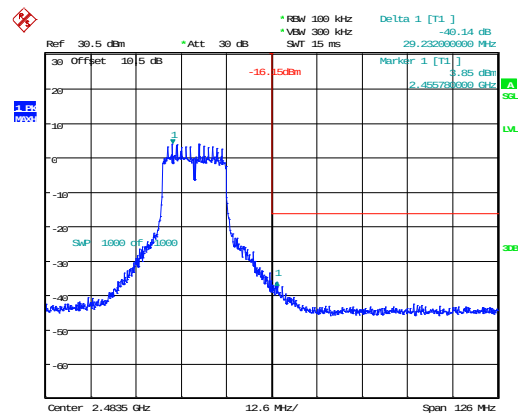
802.11n20_2462MHz
