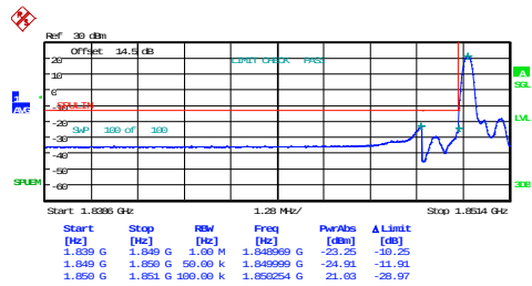
1.4MHz_Low_QPSK_1@0
