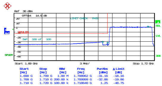
10MHz_Low_16QAM_50@0
