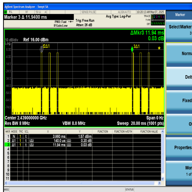
NTNV-SRD-Ant1-2439
