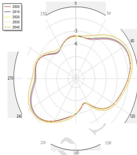
H Theta=90
