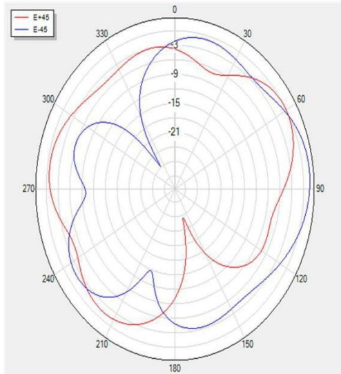
H Theta=90 freq=2400MHz
