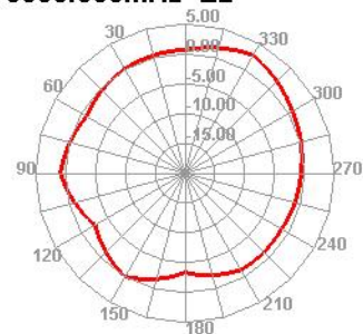
5850.000MHz E2
