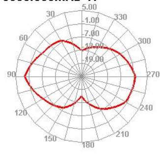
5850.000MHz H
