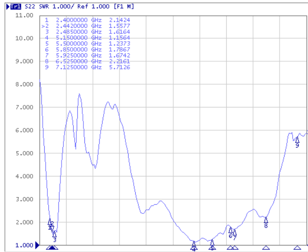
VSWR
