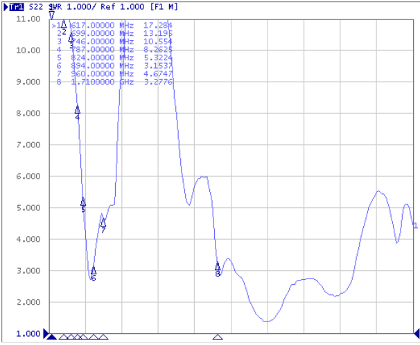
VSWR _ Low
