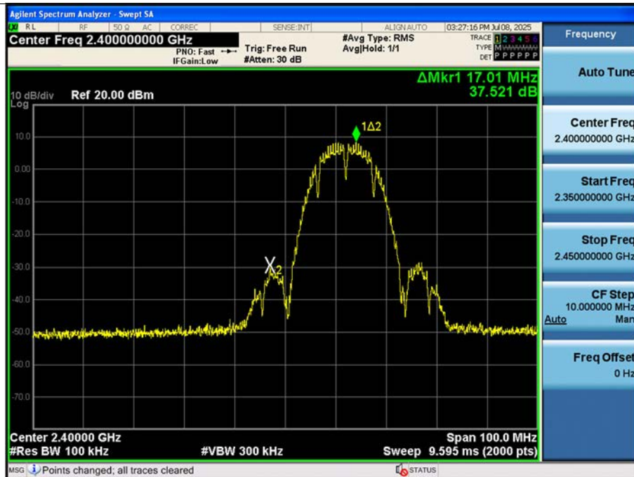
[ANT. 2] 802.11b - CH 1
