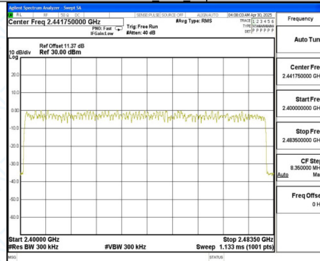
3DH5_Ant1_Hop
