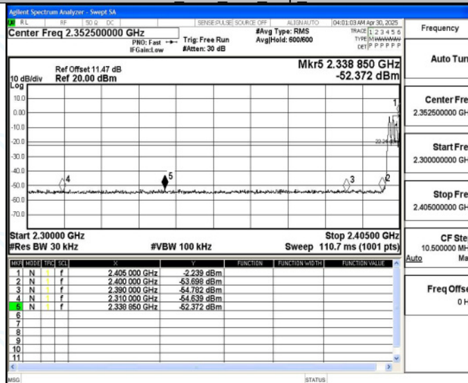
DH5_Ant1_Low_Hop_2402
