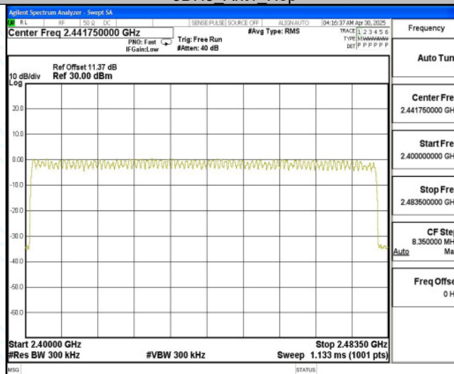
3DH5_Ant1_Hop
