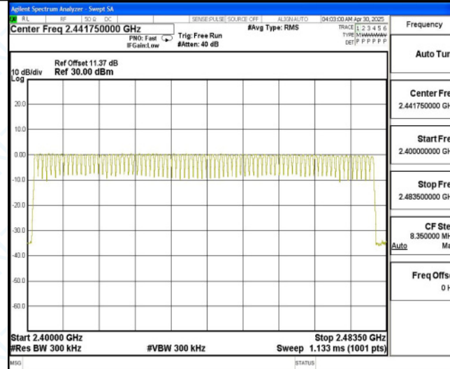
2DH5_Ant1_Hop
