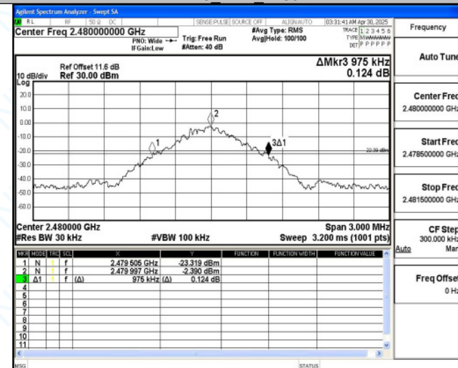
DH5_Ant1_2480
