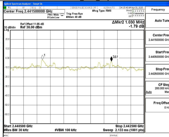
3DH5_Ant1_Hop
