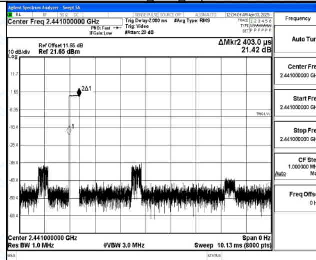
DH3_Ant1_Hop
