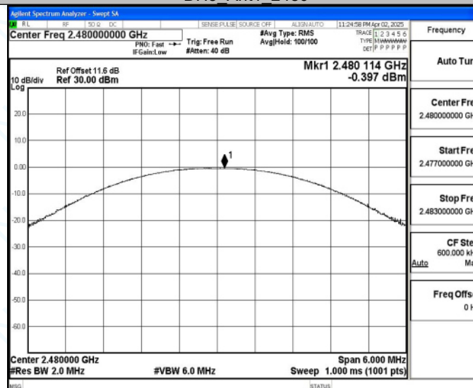
DH5_Ant1_2480
