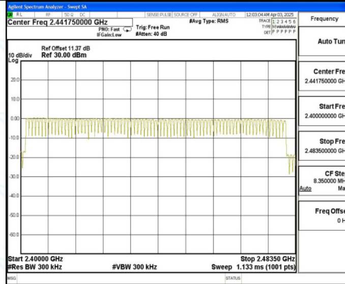
2DH5_Ant1_Hop
