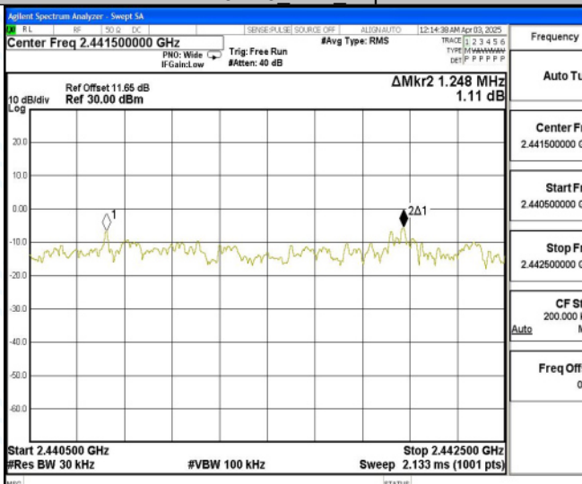
3DH5_Ant1_Hop
