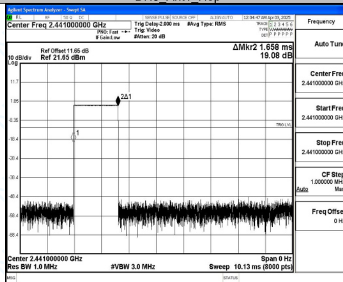
DH5_Ant1_Hop
