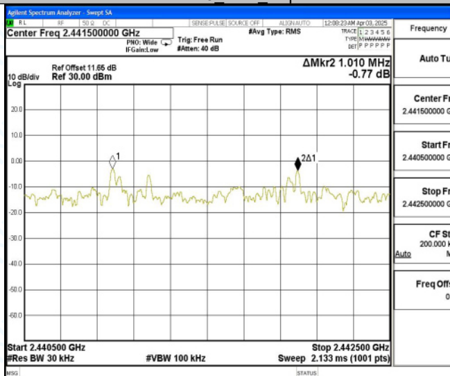
3DH5_Ant1_Hop
