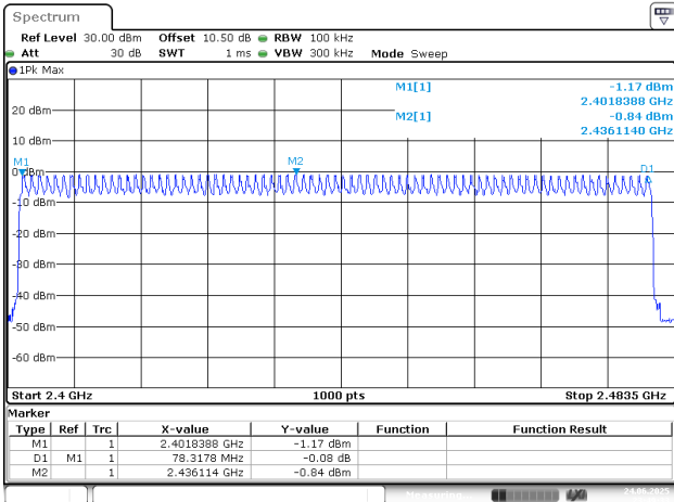
2EDR_DH1_Hopping
