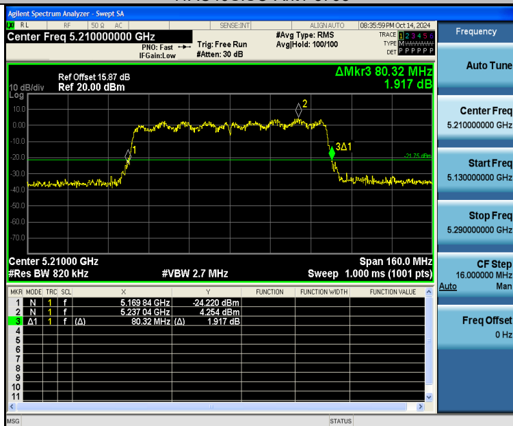
11AC80SISO-Ant1-5210
