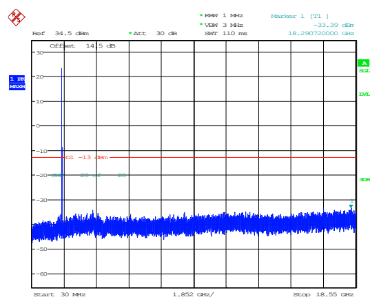
10MHz High QPSK 1@0(30MHz~18.55GHz)
