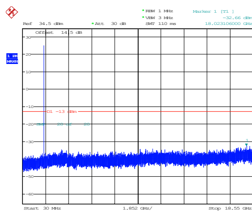
5MHz Middle QPSK 1@0(30MHz~18.55GHz)
