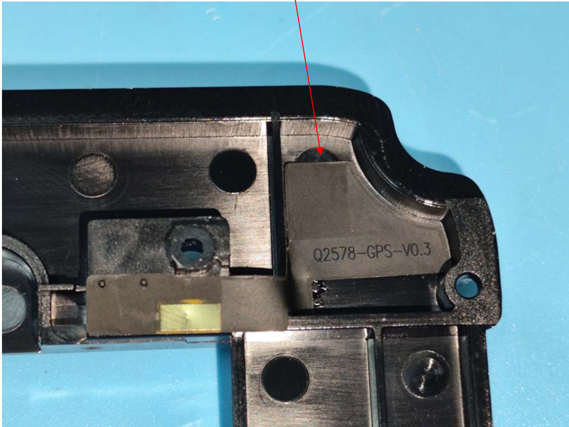
GPS Antenna
