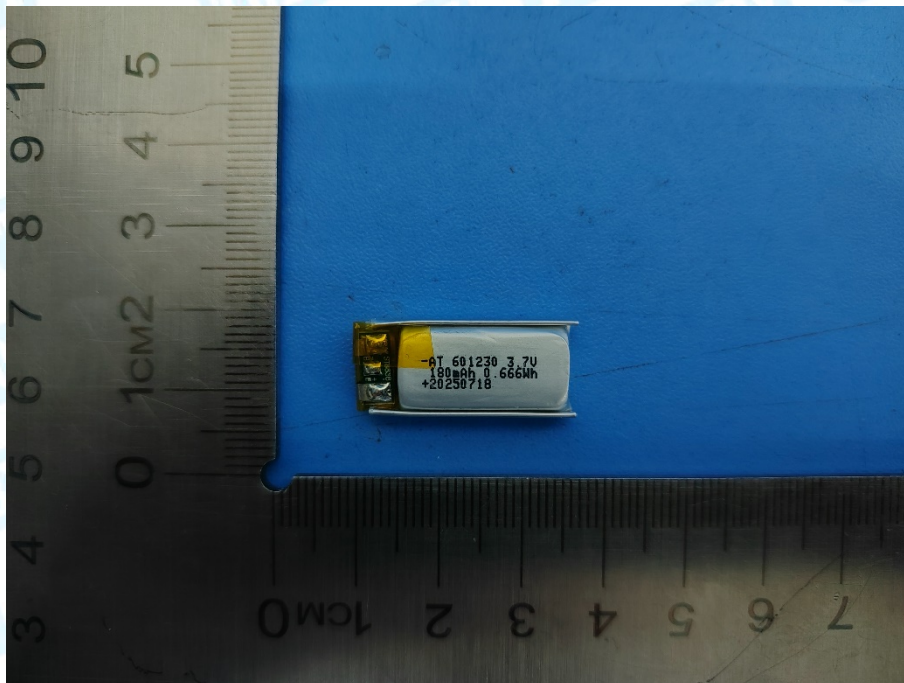
Photo 10 Battery parameters
