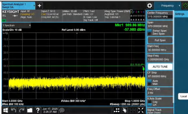
48-48-20MHz-10MHz-QPSK-QPSK-55340-55484-1RB#0-ORB#0-3 0~1000MHz-PASS
