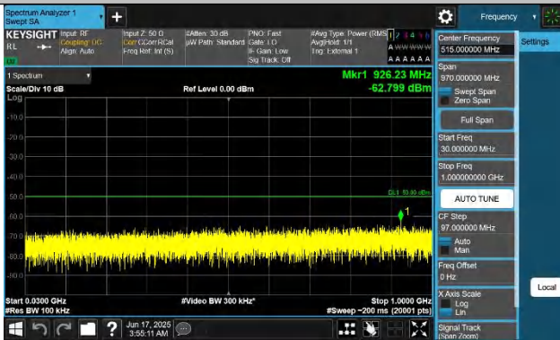
48-48-20MHz-15MHz-QPSK-QPSK-55916-56087-1RB#0-ORB#0-3 0~1000MHz-PASS
