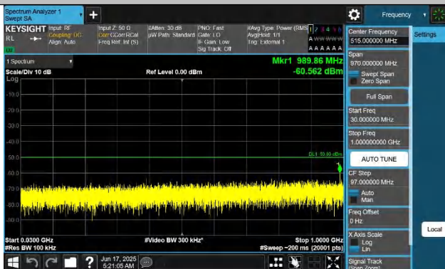
48-48-20MHz-20MHz-QPSK-QPSK-55340-55538-1RB#0-ORB#0-3 0~1000MHz-PASS
