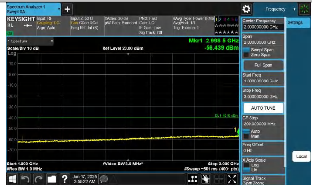
48-48-20MHz-15MHz-QPSK-QPSK-55916-56087-1RB#0-ORB#0-1 000~3000MHz-PASS
