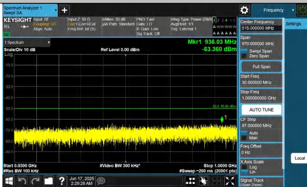
48-48-20MHz-10MHz-QPSK-QPSK-56541-56685-1RB#0-ORB#0-3 0~1000MHz-PASS
