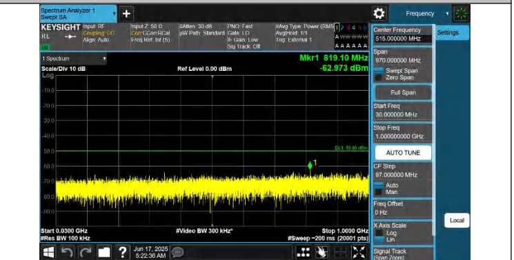
48-48-20MHz-20MHz-QPSK-QPSK-55891-56089-1RB#0-ORB#0-3 0~1000MHz-PASS
