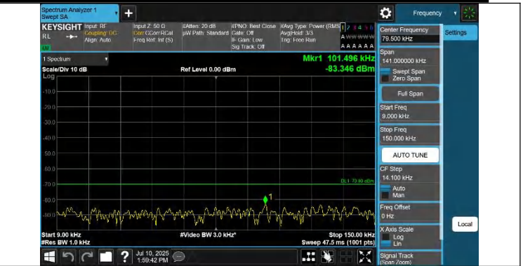
48-48-20MHz-5MHz-QPSK-QPSK-55340-55457-1RB#0-ORB#0-0. 009~0.15MHz-PASS
