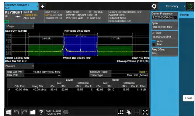
48-48-20MHz-20MHz-QPSK-QPSK-55891-56089-1RB#0-1RB#99-PASS
