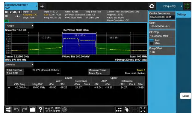
48-48-20MHz-20MHz-QPSK-QPSK-55891-56089-100RB#0-100R B#0-PASS
