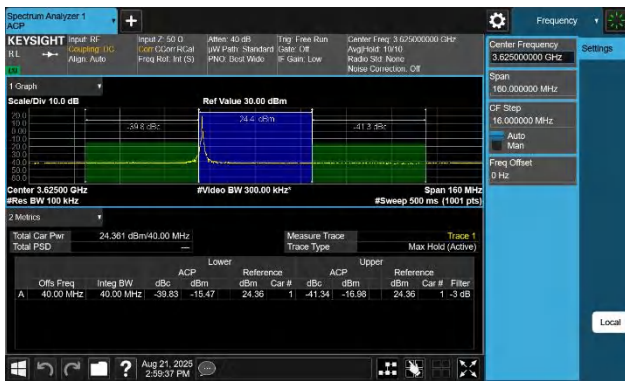
48-48-20MHz-20MHz-QPSK-QPSK-55891-56089-1RB#0-0RB#0-PASS
