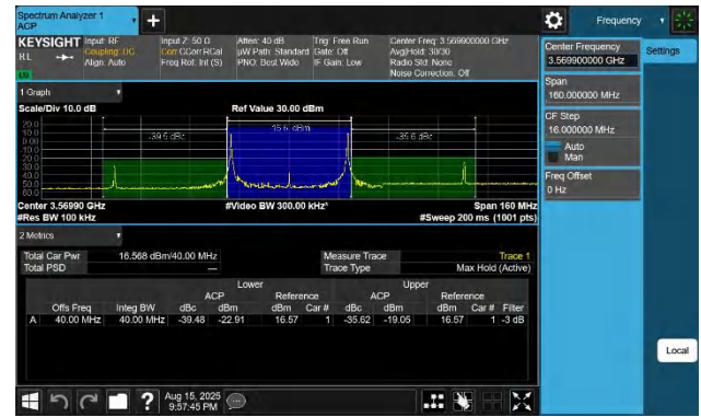
48-48-20MHz-20MHz-QPSK-QPSK-55340-55538-1RB#0-1RB#99-PASS
