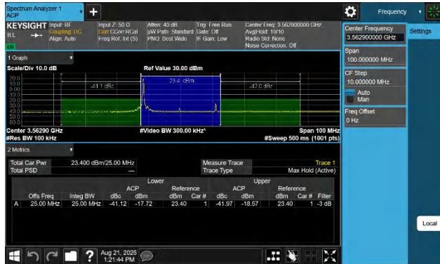
48-48-5MHz-20MHz-QPSK-QPSK-55273-55390-1RB#0-0RB#0-P ASS
