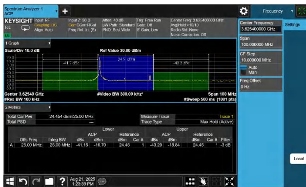
48-48-5MHz-20MHz-QPSK-QPSK-55898-56015-1RB#0-0RB#0-P ASS
