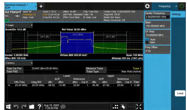
48-48-5MHz-20MHz-QPSK-QPSK-55273-55390-25RB#0-100RB# 0-PASS
