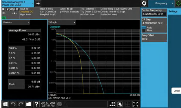
48-48-20MHz-15MHz-QPSK-QPSK-55916-56087-100RB#0-75RB#0-PASS
