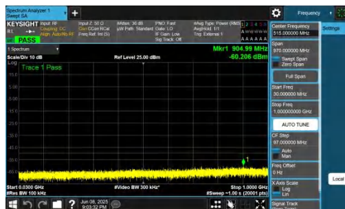
NTNV-n48-PC3-30-20-M-CP-QPSK-Inner_1RB_Left-30-1000-PA SS
