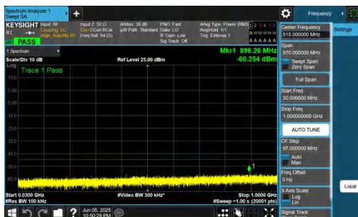
NTNV-n48-PC3-30-20-M-DFT-QPSK-Inner_1RB_Left-30-1000-PASS
