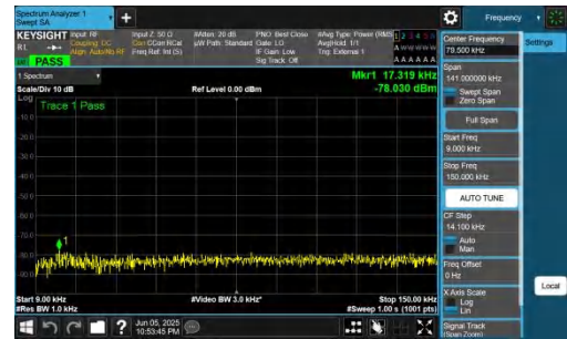
NTNV-n48-PC3-30-20-M-DFT-QPSK-Inner_1RB_Right-0.009-0.15 -PASS
