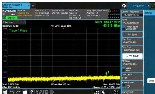
NTNV-n48-PC3-30-30-L-DFT-QPSK-Inner_1RB_Left-30-1000-PA SS
