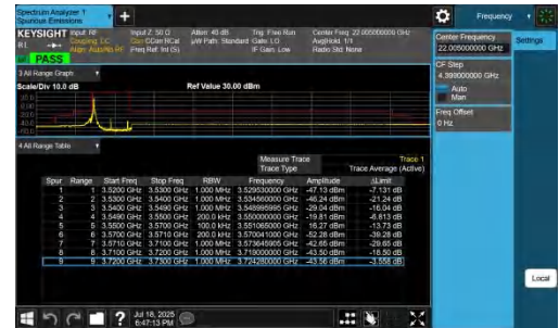
NTNV-n48-PC3-30-20-L-DFT-QPSK-Edge_1RB_Left-PASS
