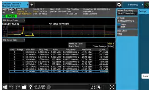
NTNV-n48-PC3-30-20-L-DFT-BPSK-Edge_1RB_Left-PASS
