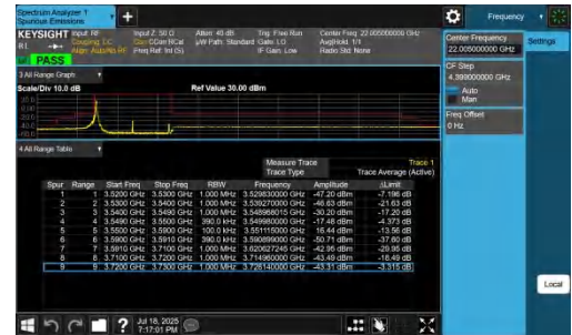
NTNV-n48-PC3-30-40-L-DFT-QPSK-Edge_1RB_Left-PASS
