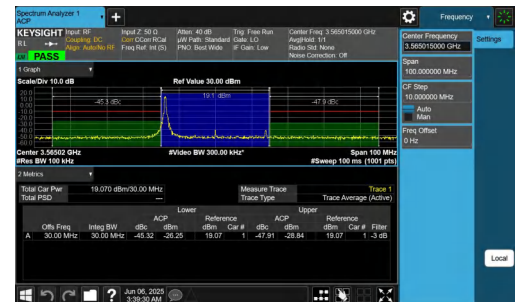
NTNV-n48-PC3-30-30-L-CP-QPSK-Edge_1RB_Left-PASS
