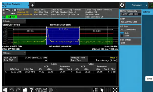
NTNV-n48-PC3-30-30-L-DFT-QPSK-Edge_1RB_Left-PASS
