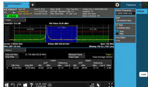
NTNV-n48-PC3-30-30-L-DFT-QPSK-Edge_1RB_Left-PASS
