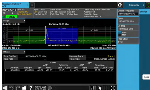
NTNV-n48-PC3-30-30-L-CP-QPSK-Edge_1RB_Left-PASS
