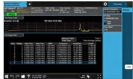
NTNV-n48-PC3-30-20-H-DFT-QPSK-Edge_1RB_Left-PASS
