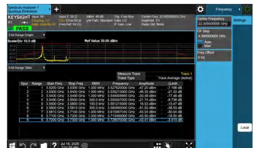
NTNV-n48-PC3-30-30-L-DFT-QPSK-Edge_1RB_Left-PASS
