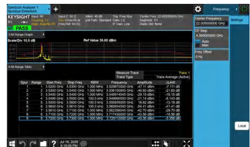
NTNV-n48-PC3-30-10-L-DFT-QPSK-Edge_1RB_Left-PASS
