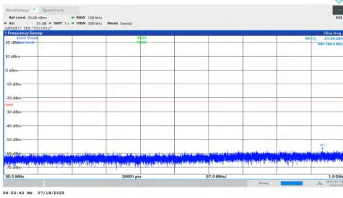
NTV-n78(3450-3550)-PC1.5-30-90-L-DFT-QPSK-Inner_1RB_Left-3 0-1000-PASS
