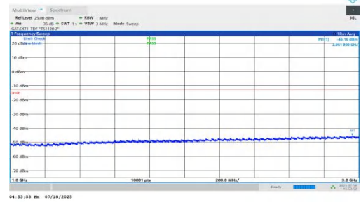
NTV-n78(3450-3550)-PC1.5-30-90-L-DFT-QPSK-Inner_1RB_Left-10 00-3000-PASS
