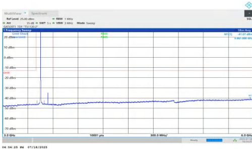
NTV-n78(3450-3550)-PC1.5-30-90-L-DFT-QPSK-Inner_1RB_Left-3 000-6000-PASS
