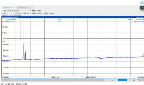
NTV-n78(3450-3550)-PC1.5-30-50-L-DFT-QPSK-Inner_1RB_Left-3 000-6000-PASS
