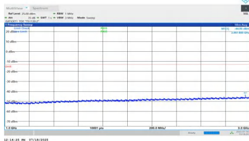
NTV-n78(3450-3550)-PC1.5-30-20-L-DFT-QPSK-Inner_1RB_Left-10 00-3000-PASS
