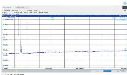
NTV-n78(3450-3550)-PC1.5-30-20-L-DFT-QPSK-Inner_1RB_Left-3 000-6000-PASS
