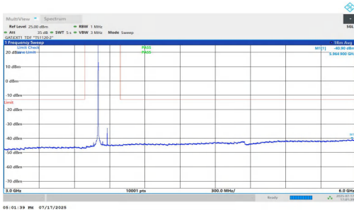
NTNV-n77(3700-3980)-PC1.5-30-80-M-DFT-QPSK-Inner_1RB_Left-3 000-6000-PASS
