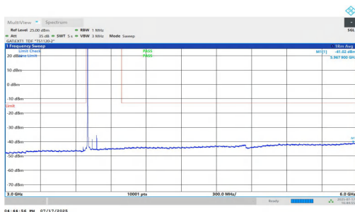
NTVN-n77(3700-3980)-PC1.5-30-80-L-DFT-QPSK-Inner_1RB_Left-3000-6000-PASS
