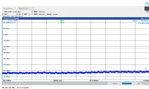
NTVN-n77(3700-3980)-PC1.5-30-80-L-DFT-QPSK-Inner_1RB_Left-30-1000-PASS
