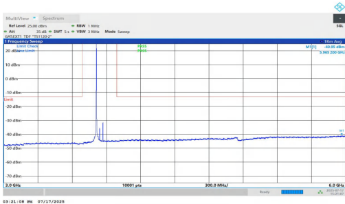
NTNV-n77(3700-3980)-PC1.5-30-60-M-DFT-QPSK-Inner_1RB_Left-3 000-6000-PASS
