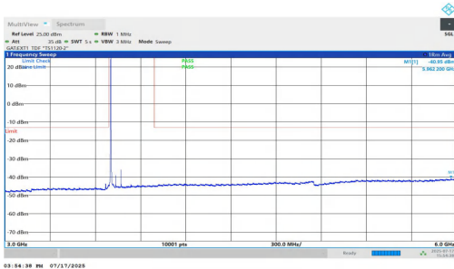
NTNV-n77(3700-3980)-PC1.5-30-70-L-DFT-QPSK-Inner_1RB_Left-3 000-6000-PASS
