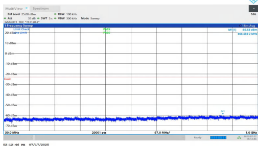
NTVN-n77(3700-3980)-PC1.5-30-50-L-DFT-QPSK-Inner_1RB_Left-3 0-1000-PASS
