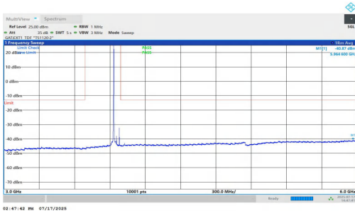
NTNV-n77(3700-3980)-PC1.5-30-50-H-DFT-QPSK-Inner_1RB_Left-3 000-6000-PASS
