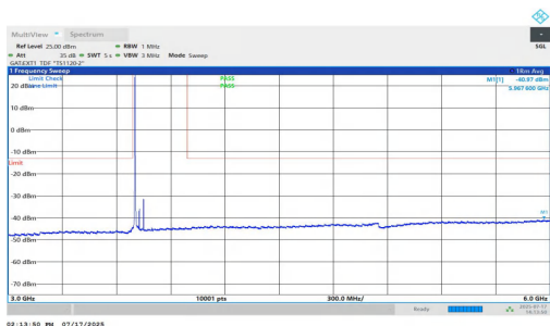
NTVN-n77(3700-3980)-PC1.5-30-50-L-DFT-QPSK-Inner_1RB_Left-3 000-6000-PASS
