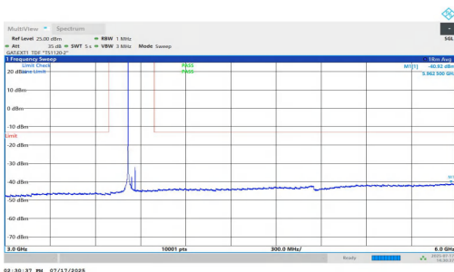
NTNV-n77(3700-3980)-PC1.5-30-50-M-DFT-QPSK-Inner_1RB_Left-3000-6000-PASS
