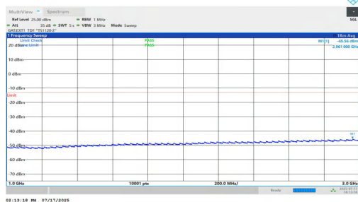
NTVN-n77(3700-3980)-PC1.5-30-50-L-DFT-QPSK-Inner_1RB_Left-10 00-3000-PASS
