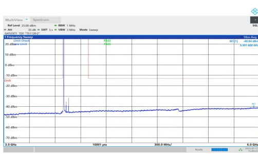
NTVN-n77(3700-3980)-PC1.5-30-60-L-DFT-QPSK-Inner_1RB_Left-3000-6000-PASS
