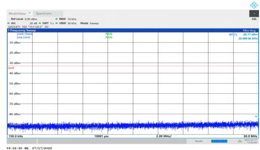
NTVN-n77(3700-3980)-PC1.5-30-60-L-DFT-QPSK-Inner_1RB_Left-0.15-5-30-PASS
