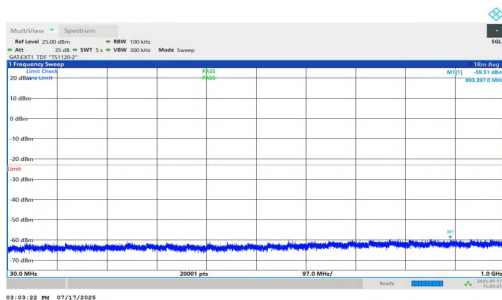
NTVN-n77(3700-3980)-PC1.5-30-60-L-DFT-QPSK-Inner_1RB_Left-30-1000-PASS
