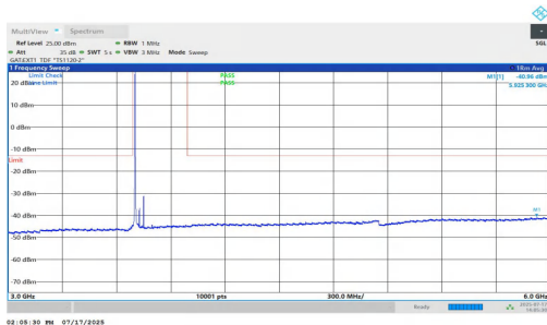
NTV-n77(3700-3980)-PC1.5-30-50-L-DFT-BPSK-Inner_1RB_Left-3000-6000-PASS
