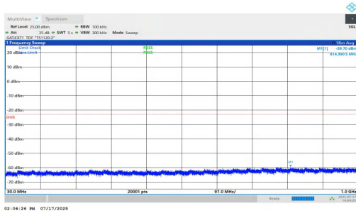
NTV-n77(3700-3980)-PC1.5-30-50-L-DFT-BPSK-Inner_1RB_Left-30-1000-PASS
