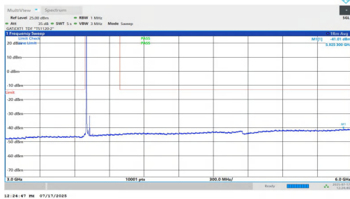
NTV-n77(3700-3980)-PC1.5-30-30-L-DFT-BPSK-Inner_1RB_Left-3000-6000-PASS
