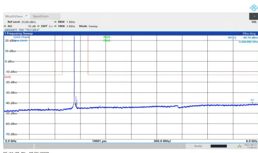
NTNV-n77(3700-3980)-PC1.5-30-25-M-DFT-QPSK-Inner_1RB_Left-3 000-6000-PASS
