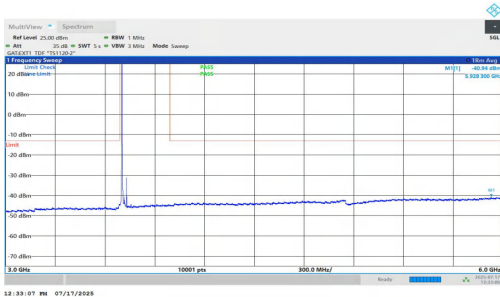
NTVN-n77(3700-3980)-PC1.5-30-30-L-DFT-QPSK-Inner_1RB_Left-3 000-6000-PASS
