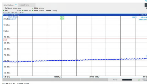
NTNV-n77(3700-3980)-PC1.5-30-25-M-DFT-QPSK-Inner_1RB_Left-10 00-3000-PASS
