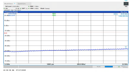
NTVN-n77(3700-3980)-PC1.5-30-30-L-DFT-QPSK-Inner_1RB_Left-10 00-3000-PASS
