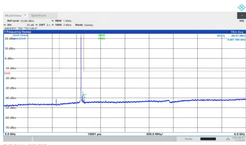
NTNV-n77(3700-3980)-PC1.5-30-25-H-DFT-QPSK-Inner_1RB_Left-3000-6000-PASS
