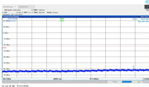
NTV-n77(3700-3980)-PC1.5-30-20-L-DFT-BPSK-Inner_1RB_Left-30-1000-PASS
