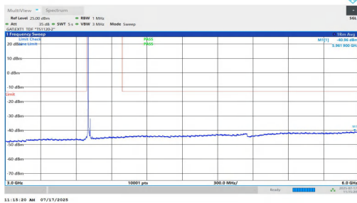
NTV-n77(3700-3980)-PC1.5-30-20-L-DFT-BPSK-Inner_1RB_Left-3000-6000-PASS
