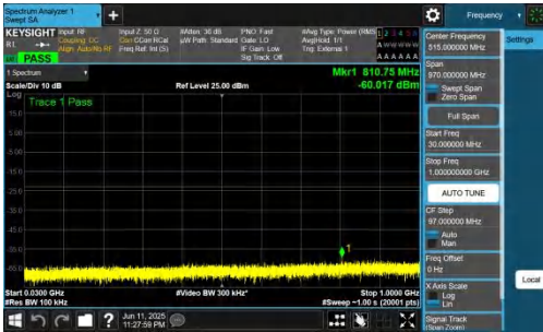
NTNV-n77(3700-3980)-PC2-30-25-M-DFT-QPSK-Inner_1RB_Left-30-1000-PASS
