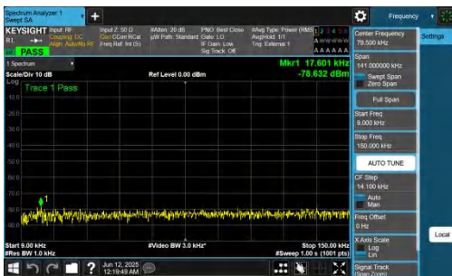
NTVN-n77(3700-3980)-PC2-30-30-M-DFT-QPSK-Inner_1RB_Left-0.09-PASS
