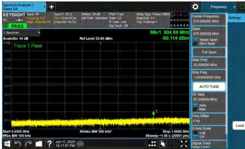
NTNV-n77(3700-3980)-PC2-30-20-L-DFT-QPSK-Inner_1RB_Left-30-1000-PASS
