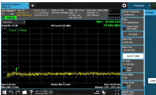
NTNV-n77(3700-3980)-PC2-30-20-M-DFT-QPSK-Inner_1RB_Left-0.09-PASS
