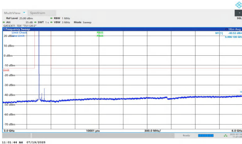
NTVN-n77(3450-3550)-PC1.5-30-70-L-DFT-QPSK-Inner_1RB_Left-3 000-6000-PASS
